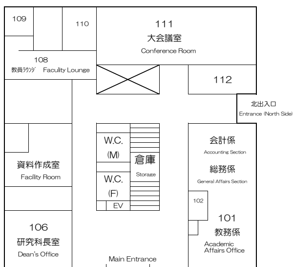
1階
